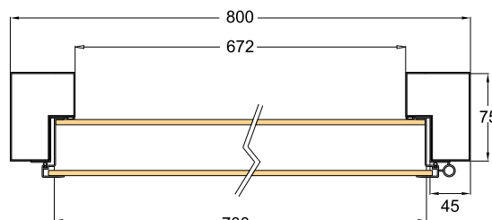
Cerradura vista interior
