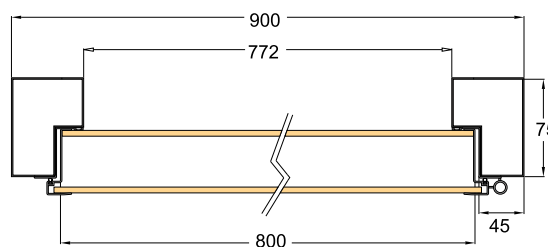
Rejilla de ventilación (opcional)
